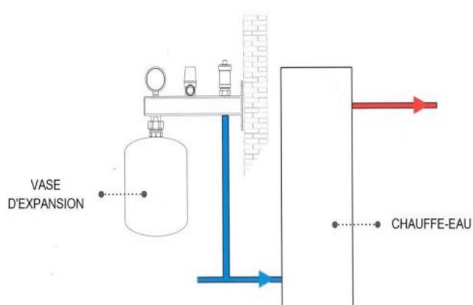
MONTAGE SUR UNE INSTALLATION AVEC CHAUFFE-EAU
