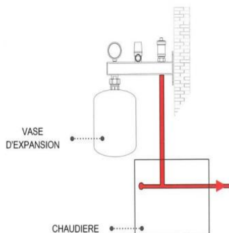
MONTAGE SUR UNE INSTALLATION AVEC CHAUFFAGE CENTRAL
